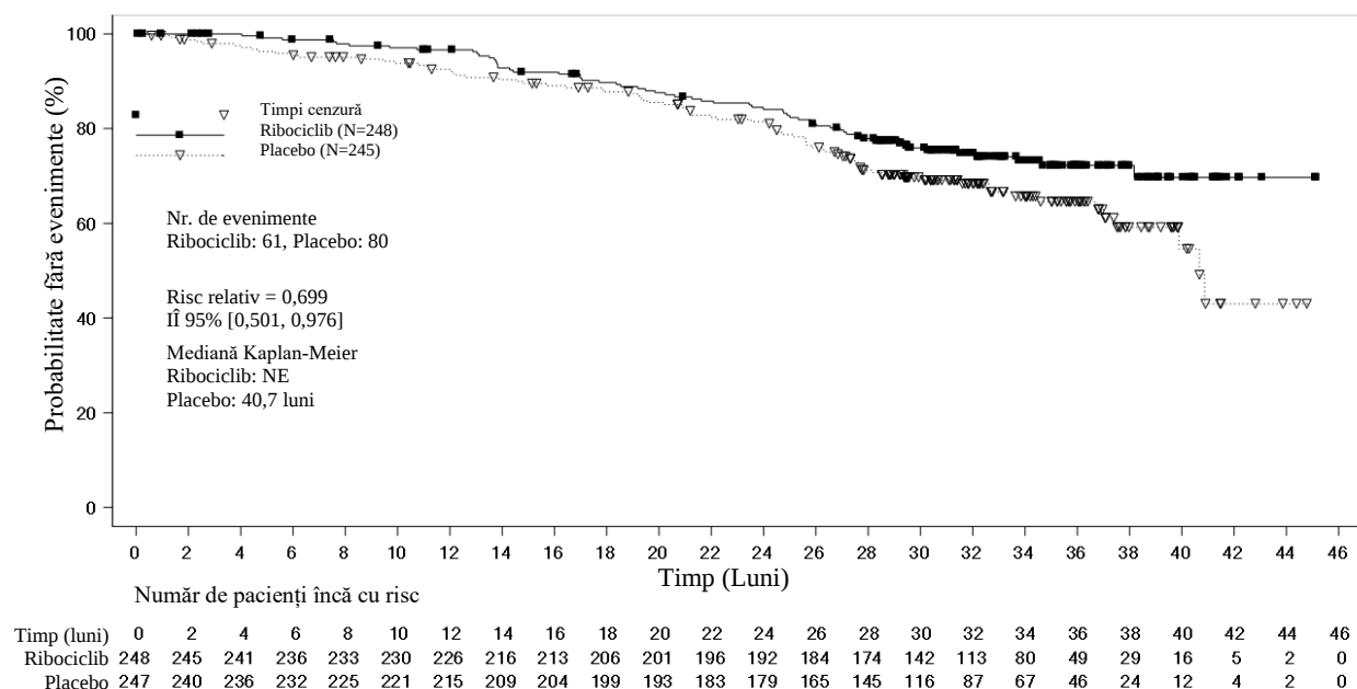
Figura 7 MONALEESA-7 – Grafic Kaplan Meier al analizei SG finale la pacienții care au administrat IANS (data centralizării 30 noiembrie 2018)
